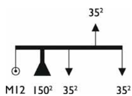
Schéma grille d'étoilement IP2X
