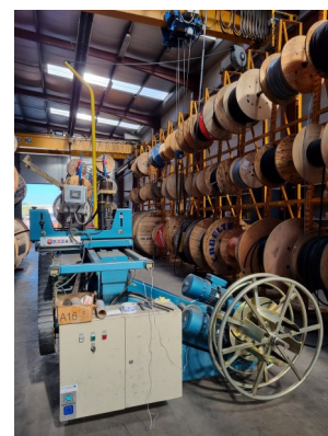
6 racks à câbles et 3 enrouleuses-couronneuses
